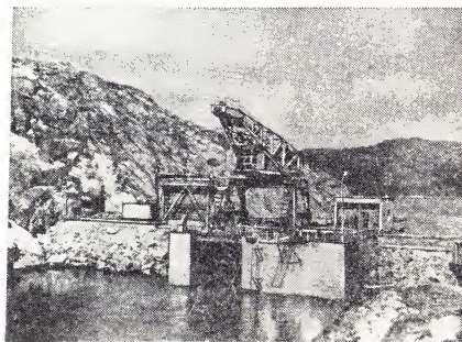
Рис. 3. Кислогубская ПЭС (СССР), вид с моря.
